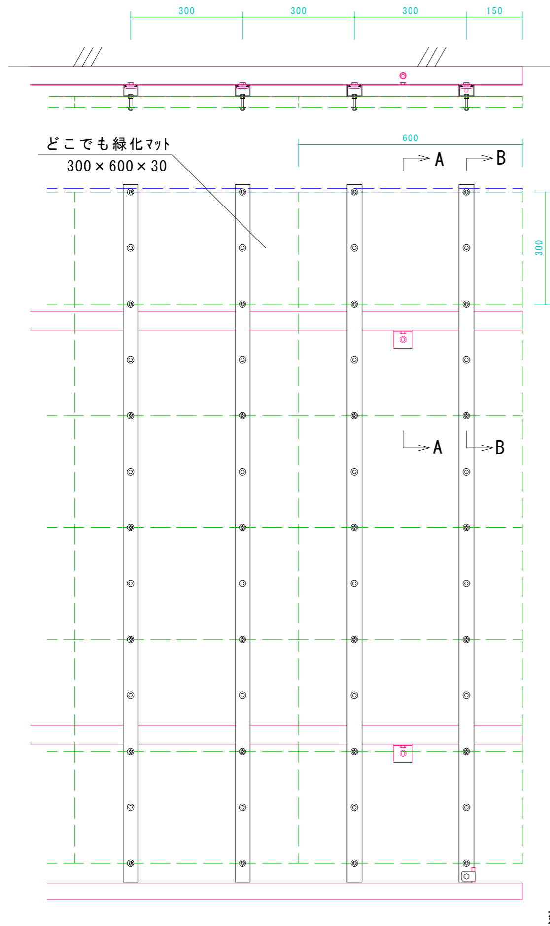
正面 S=1/10
