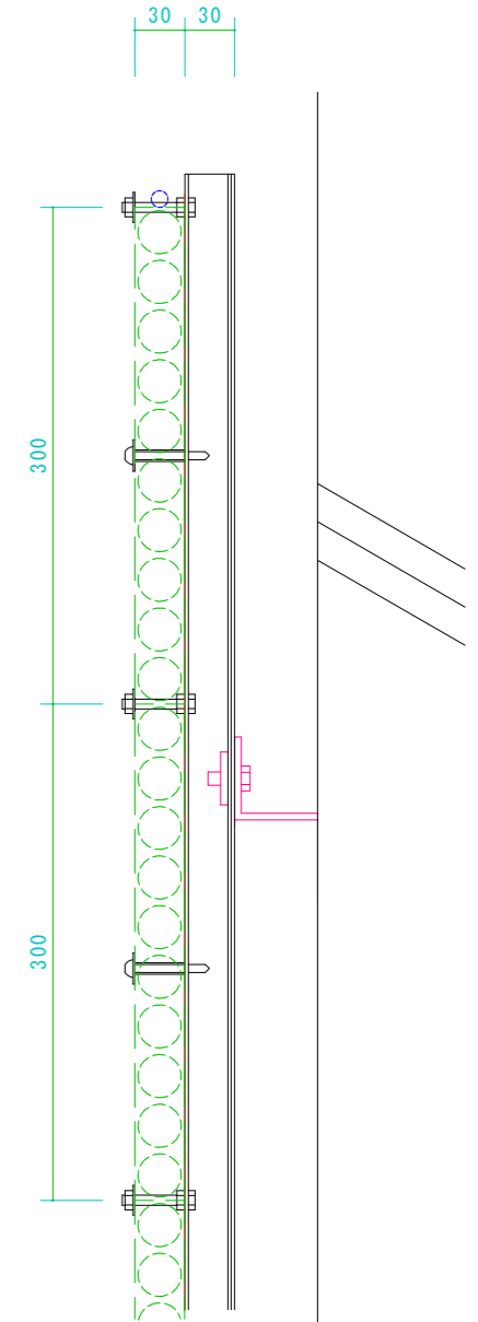
B-B断面 S=1/5
