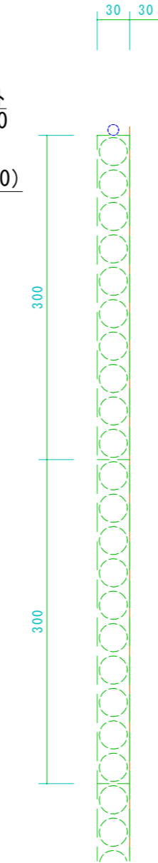
A-A断面 S=1/5
